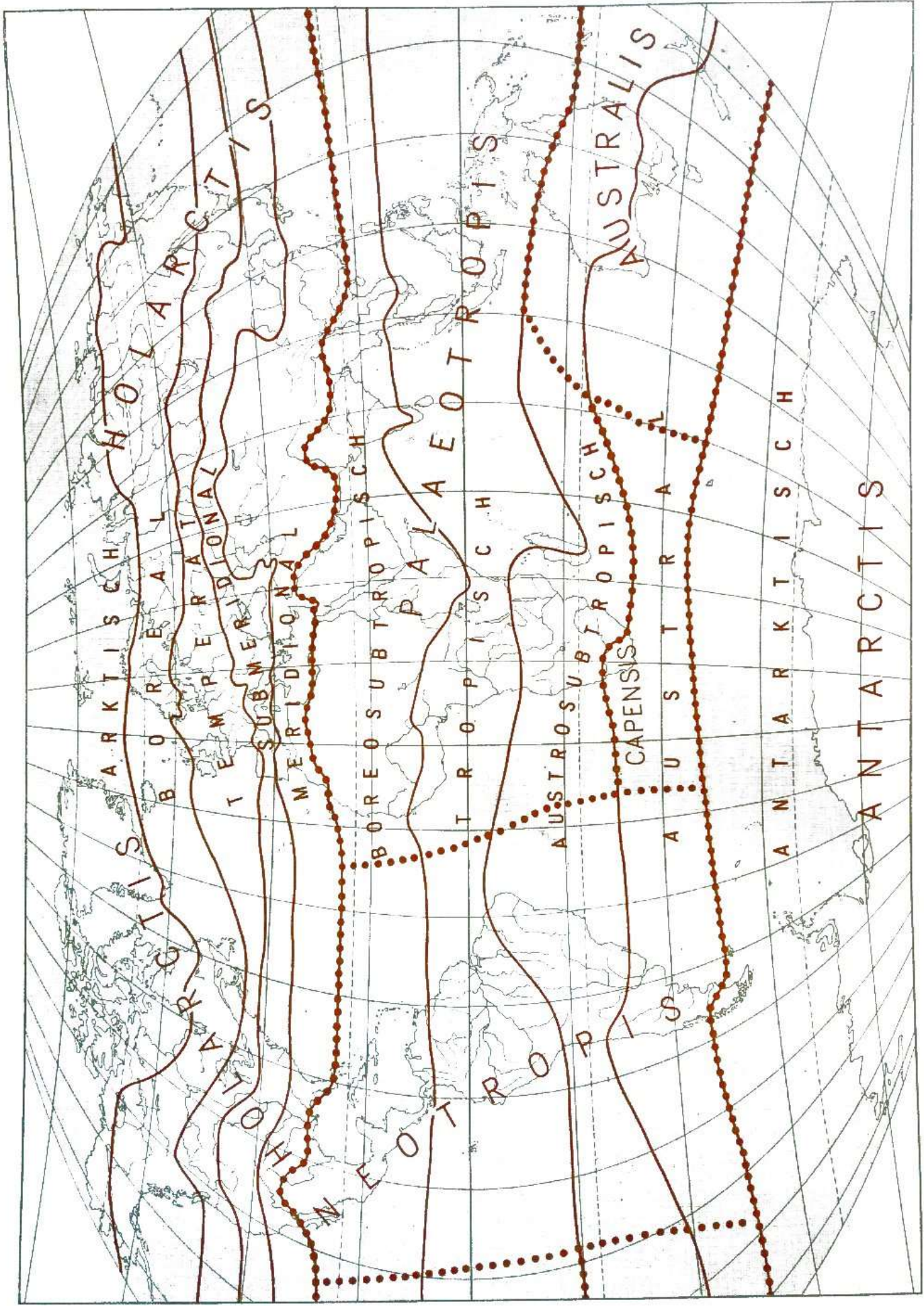
Florenreiche und Florenzonen der Erde
